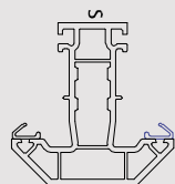
702503 70mm T Transom
