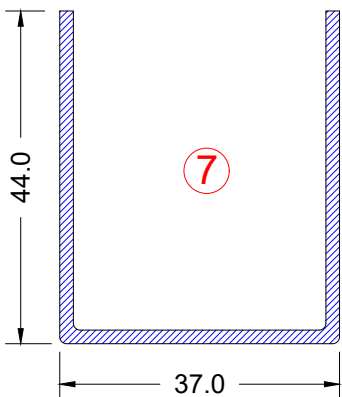
Door sash
