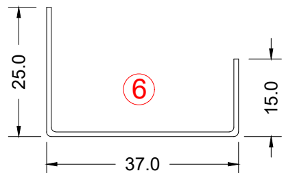
T/T sash
