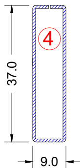
transom
