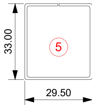
Door Outer
