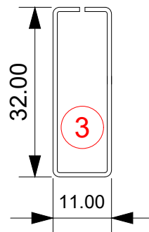
Transom
