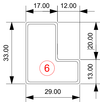
Door Outer
