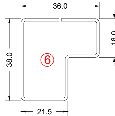
Door Outer
