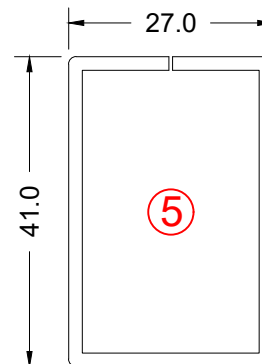
Door Mullion
