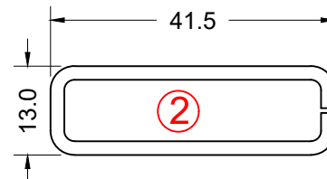
Door Mullion
