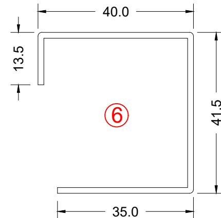
Door Sash
