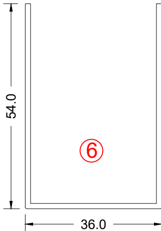
Door Sash
