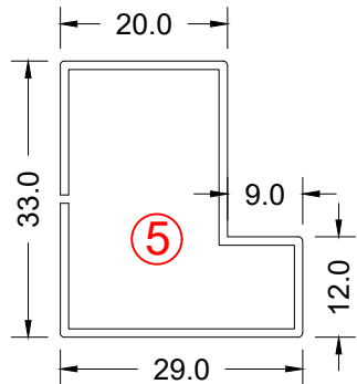
Door Frame
