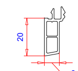
110.104 20mm Odd Leg/Drip
